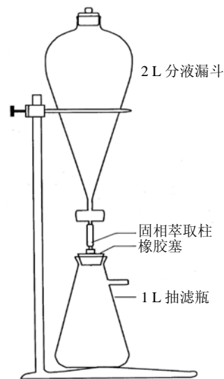
图 1 固相萃取装置 (萃取部分) 示意图
